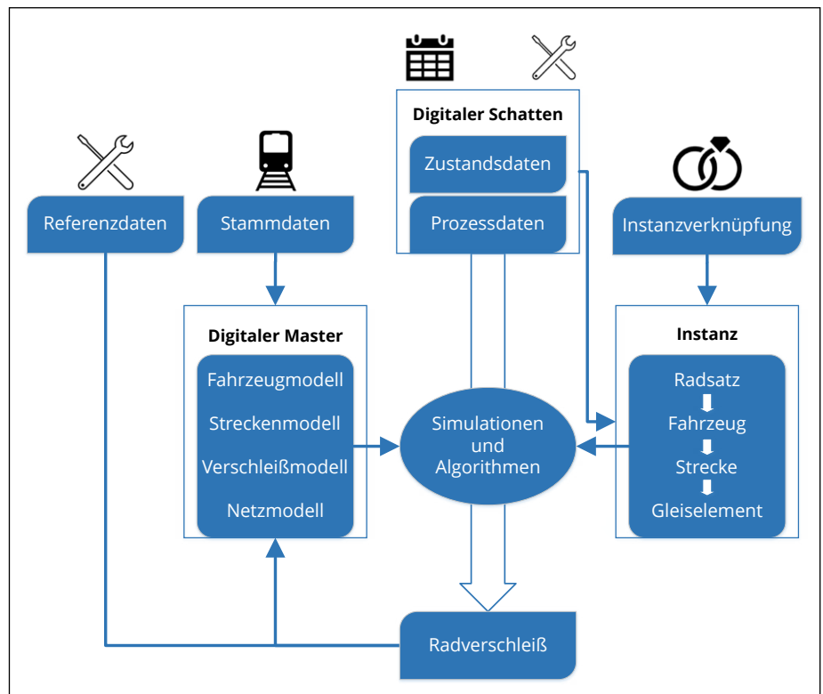
Abb. 3: Konzeptskizze des Digitalen Zwillinges zur Radverschleißprognose
