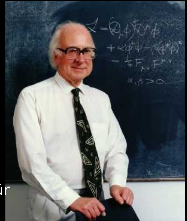
Peter Ware Higgs (* 29.05.1929)
