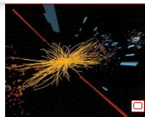
Simulation eines möglichen Zerfalls eines Higgs-Bosons. Foto: dpa
